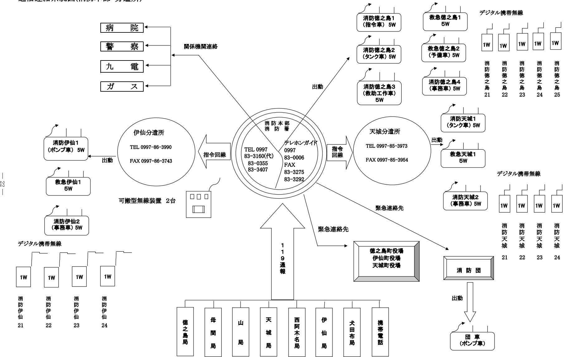
通信連絡系統図(消防本部・分遣所)
